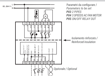
Fig. 1: Schema di collegamento per un impianto a 2 tubi con pilotaggio di una valvola on/off caldo/freddo e un ventilatore AC a tre velocità. Wiring diagram for a 2-pipes system with an on/off hot/cold valve and a three-speeds AC fan motor.
