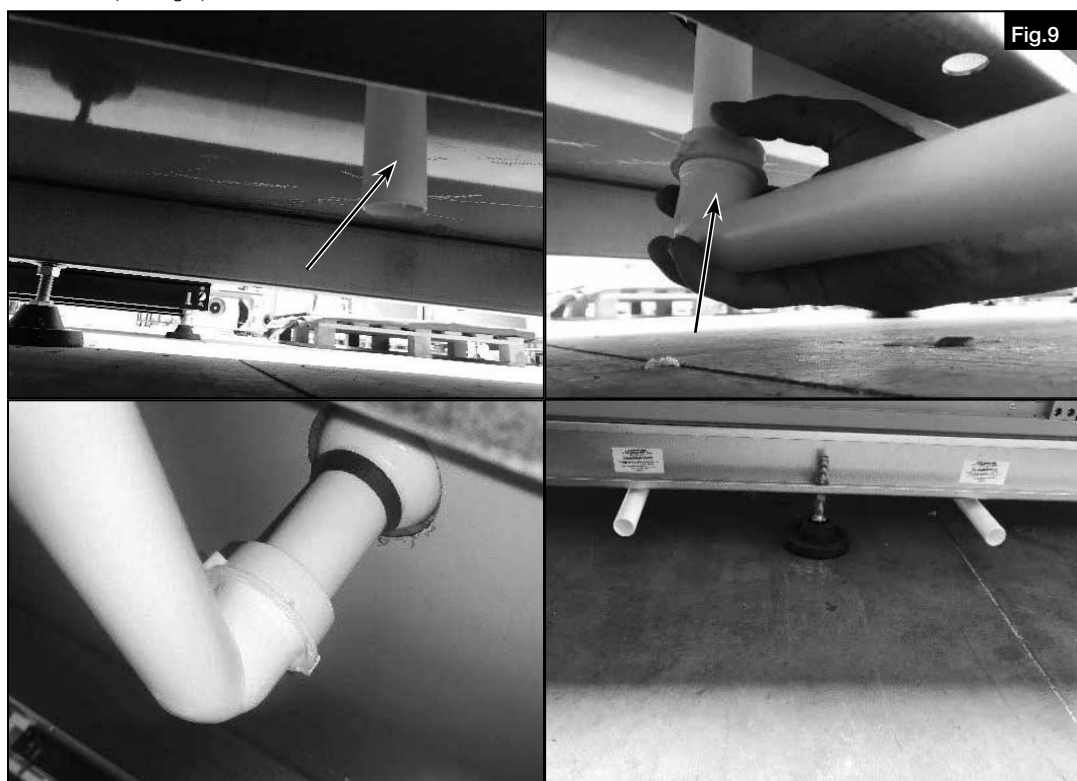
2. Fixer le coude du conduit sous le bac à condensat. S'assurer que la construction est étanche en faisant tourner le raccord (voir Fig.9).
