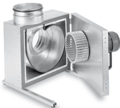
Mega Box met voorwaarts gekromd schoepenwiel
