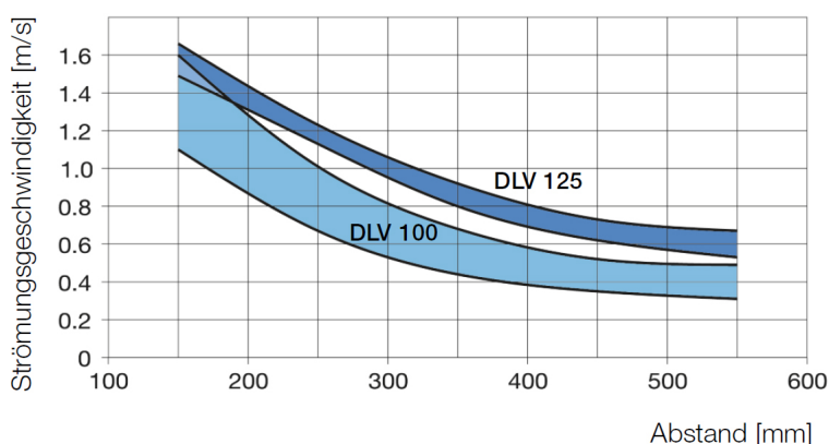
DLV 100 – DLV 125
