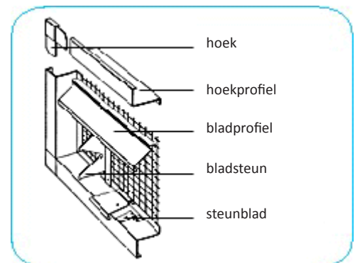
HOEK BR 40 Alumir
